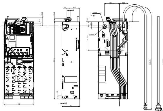
CL-T100安装尺寸
